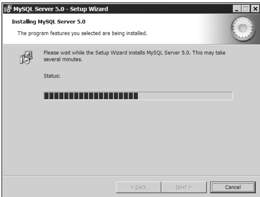
Рис. 1.7. Копирование файлов
