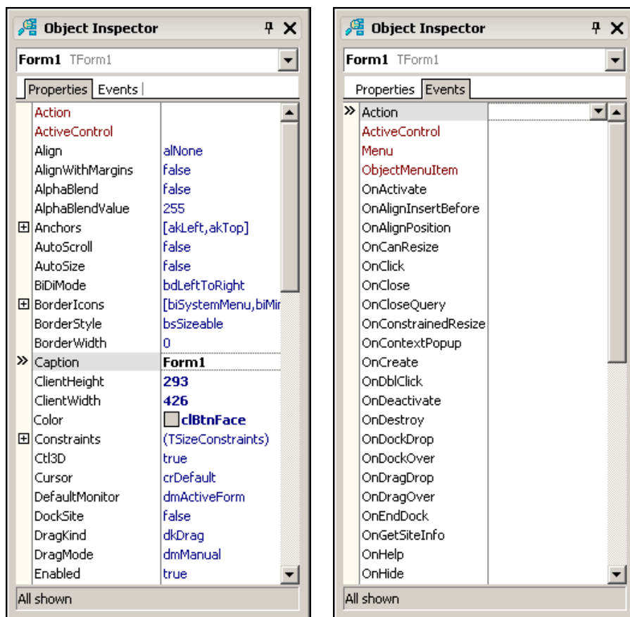
Рис. 1.4. В окне Object Inspector на вкладке Properties перечислены свойства объекта, а на вкладке Events — события, на которые объект может реагировать
