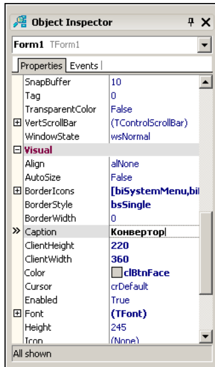
Рис. 2.2. Изменение значения свойства Caption путем ввода нового значения
