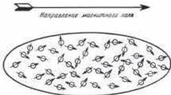
Рис. 1. Парамагнетизм
