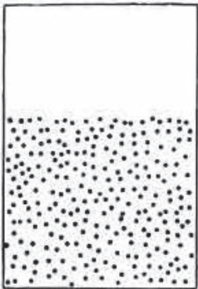
Рис. 2. Оседающий туман
