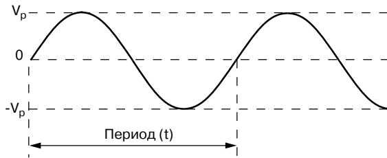
Рис. 1.1. Синусоидальная волна
