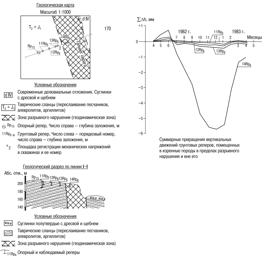
Рис. 2. Инструментальные наблюдения сдвижения реперов на Южном берегу Крыма
