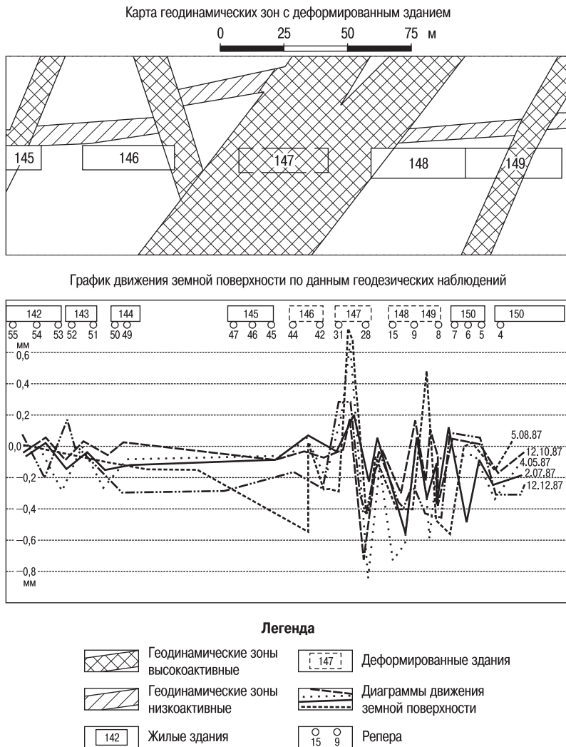
Рис. 4. Результаты геодезических наблюдений в районе геодинамической зоны (Донбасс)
