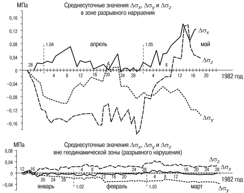
Рис. 3. Тензометрические наблюдения в зоне разрывного нарушения и вне его (ЮБК)
