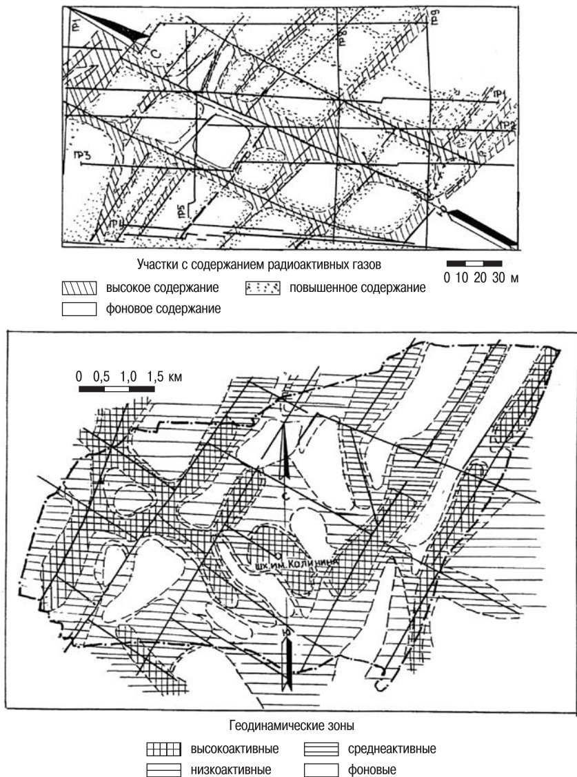
Рис. 1. Геодинамические карты участков строительства лабораторного корпуса ЦОНТБ и шахтного поля им. Калинина в г. Донецке
