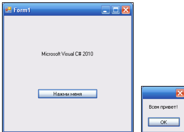
Рис. 1.6. Работающая программа
