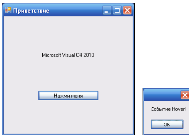
Рис. 1.7. Работа программы
