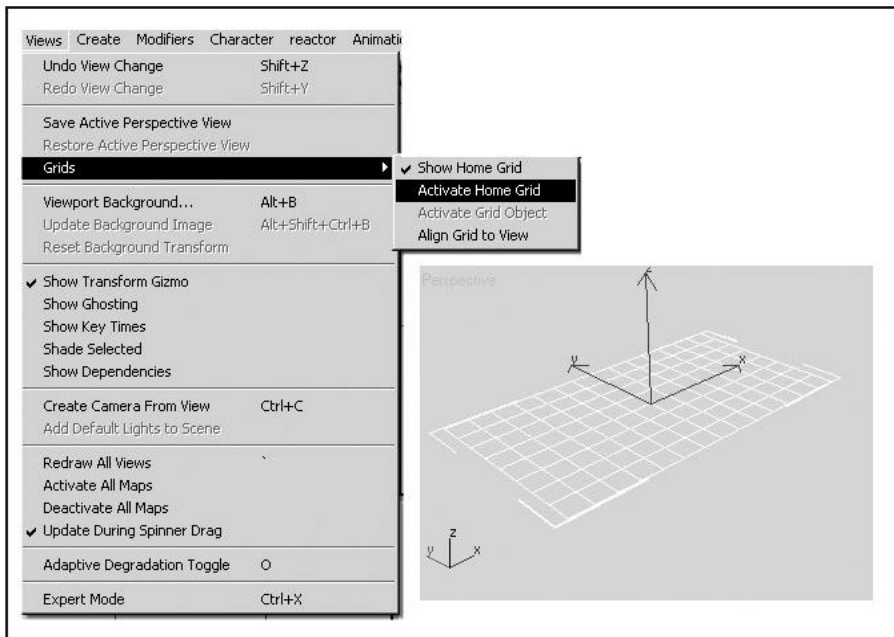
Рис. 2.12. Активизация объекта-сетки
