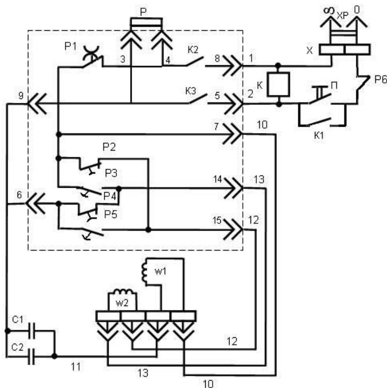
Рисунок 2.4 - Стиральная машина типа СМР
