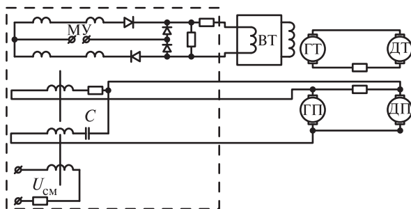
Рис. 1.4. Схема автоматического подъема ковша к месту разгрузки: МУ — магнитный усилитель; ВТ — возбудитель привода тяги; ГТ, ГП, ДТ, ДП — генератор, двигатель приводов подъёма и тяги; U_{см} — напряжение смещения
