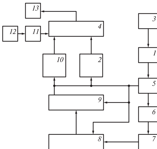
Рис. 1.5. Блок-схема устройства автоматического транспортирования ковша драглайна:
