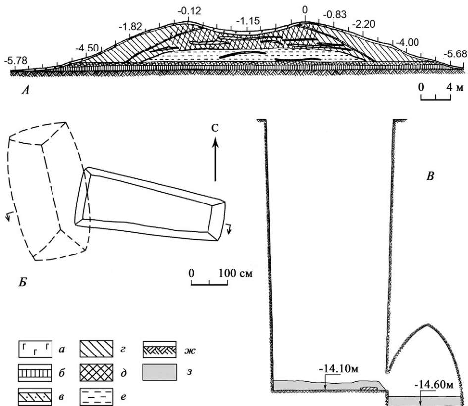
Рис. 2. Андрейаульский курганный могильник. Курган 1. Профиль северной стенки траншеи (А), план (Б) и разрез (В) катакомбы (по: Магомедов, 1987)
