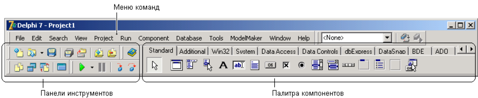
Рис. 1.7. Главное окно
